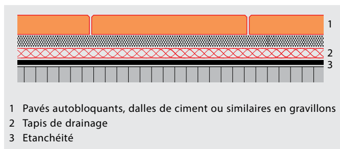
Fig. 4: structure d'un système de couche d'usure fermée sur une construction à toit plat isolée thermiquement.
